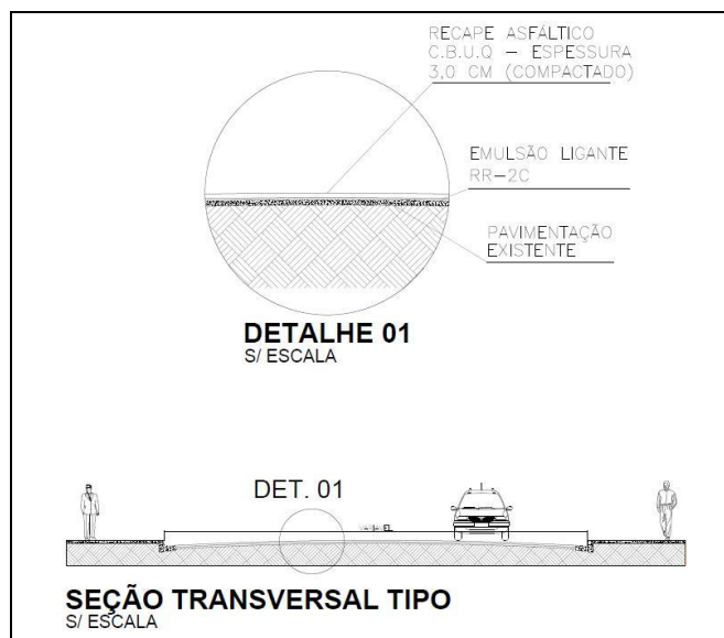
Imagem 05. Detalhe e Seção Transversal Tipo.
